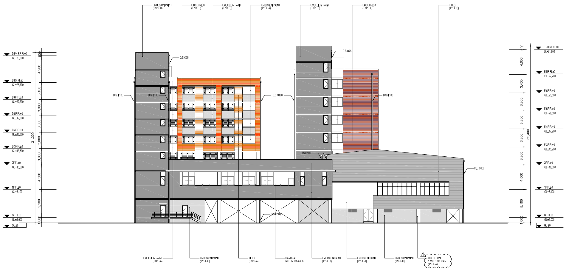
1 WEST ELEVATION SCALE: A1 1/150 A3 1/300
