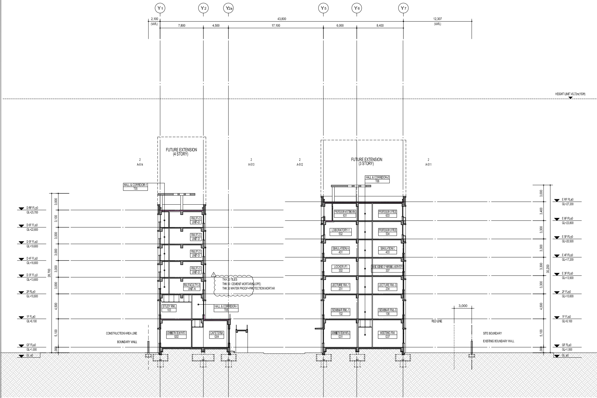
1 D - D' SECTION SCALE: A1 1/150 A3 1/300
