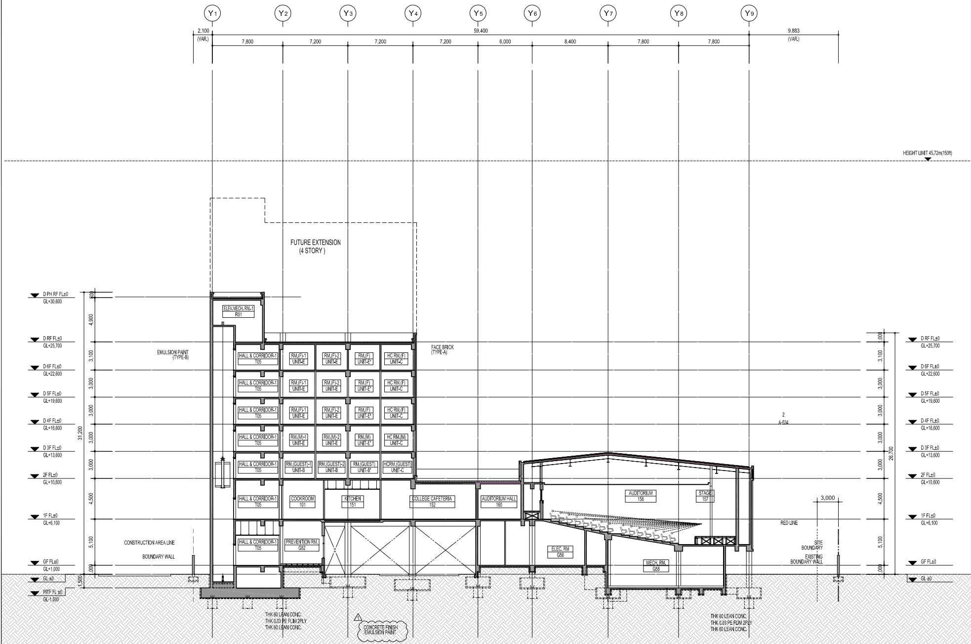
1 C - C' SECTION SCALE: A1 1/150 A3 1/300
