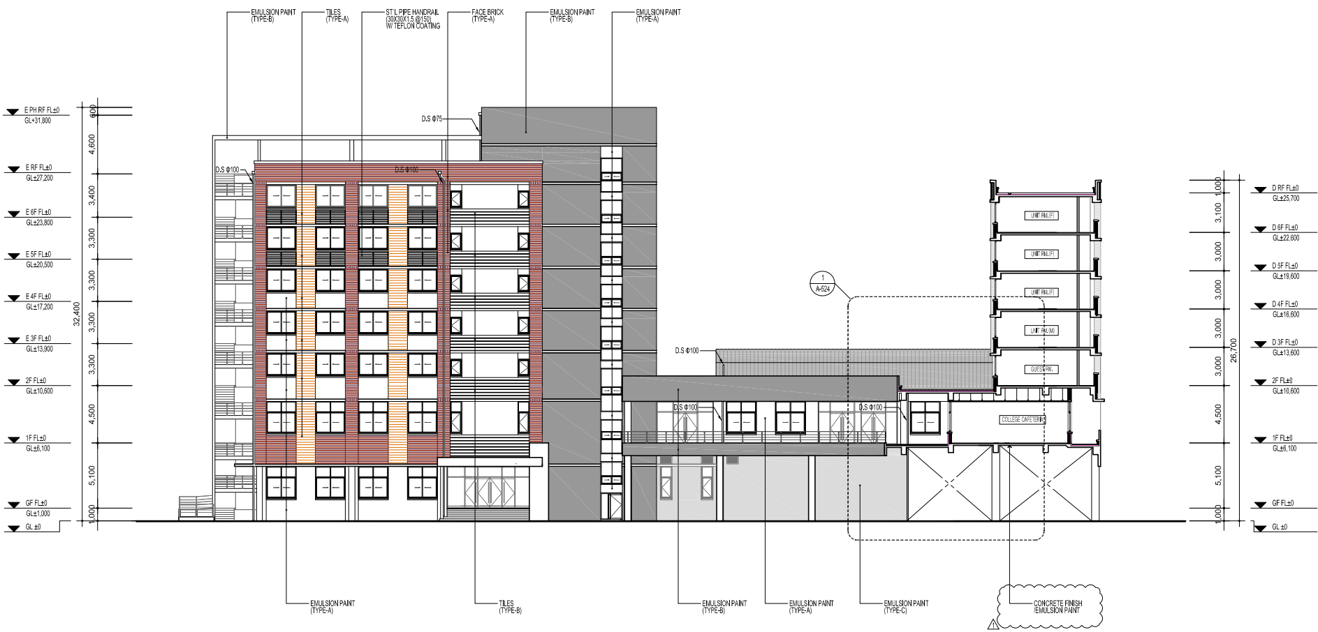
1 NORTH ELEVATION - 2 SCALE: A1 1/150 A3 1/300
