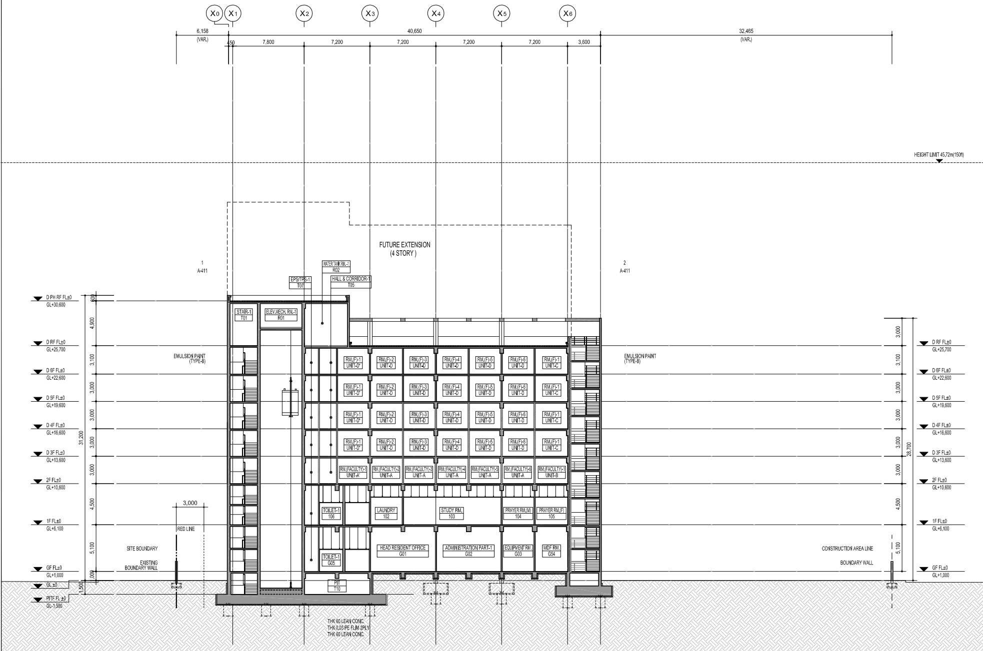
A - A' SECTION SCALE: A1 1/150 A3 1/300
