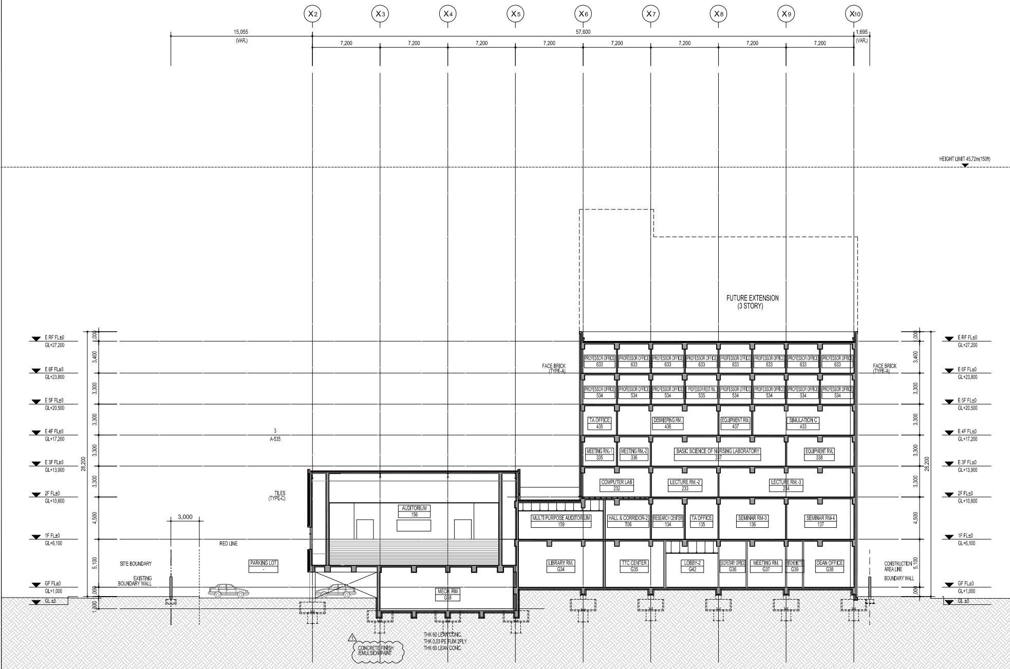
B - B' SECTION SCALE: A1 1/150 A3 1/300
