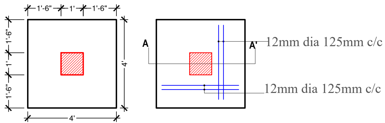
F1C1 PLAN
